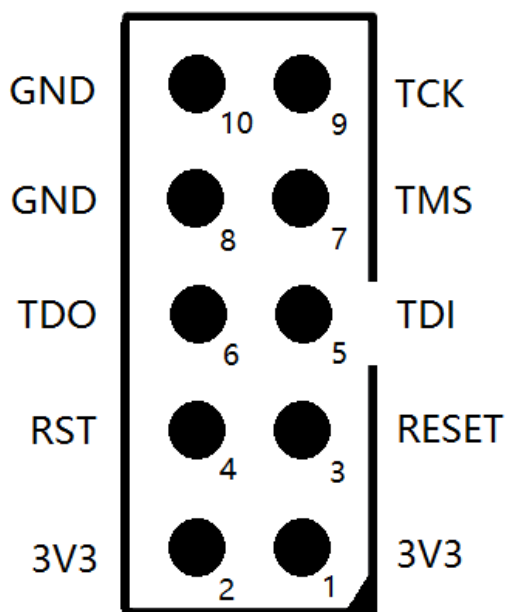
XDS110 引脚排列
